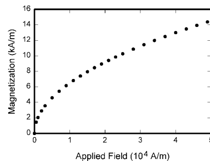
ภาพที่ 1 แสดงความสัมพันธ์ระหว่าง Applied Field กับ Magnetization ของวัสดุชนิด XYZ (ภาพที่....จะอยู่ด้านล่างของภาพ)
